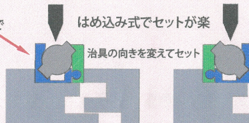
円形斜め及び側面部のディンプルをカットする(BT-1 治具 Bを使用) 治具の向きを変えてセット
